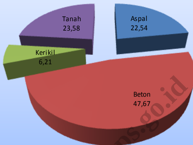
Gambar 8.1 Panjang Jalan Menurut Jenis Permukaan Tahun 2013 Length of Roads by Surface, 2013 (%)
